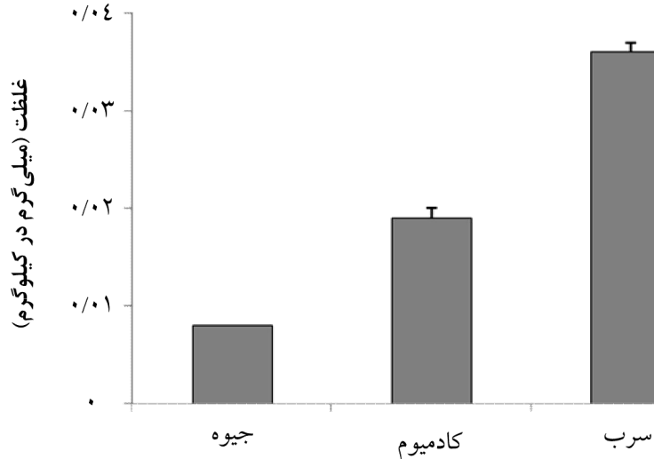
شکل ۱- میزان فلزات سنگین جیوه، کادمیوم و سرب (میلی‌گرم در کیلوگرم) در تخم ماهی قزل‌آلای رنگین‌کمان ( Oncorhynchus mykiss )
